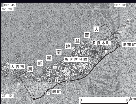
人吉盆地南縁断層 (地震調査研究推進本部 HP より)
