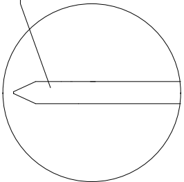
B部(矢じり加工) 詳細図
